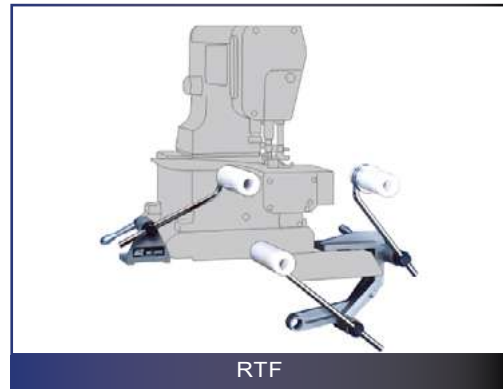
Burunlu Reçme Lastik Gerdirci (Mekanik)
