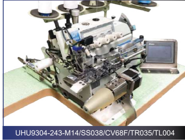
Full Otomatik 4 İplik Yaka Takma Overlok Otomatı
