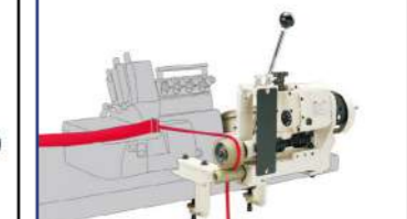
Overloklar için Önden Çekici (Spagetti için)
